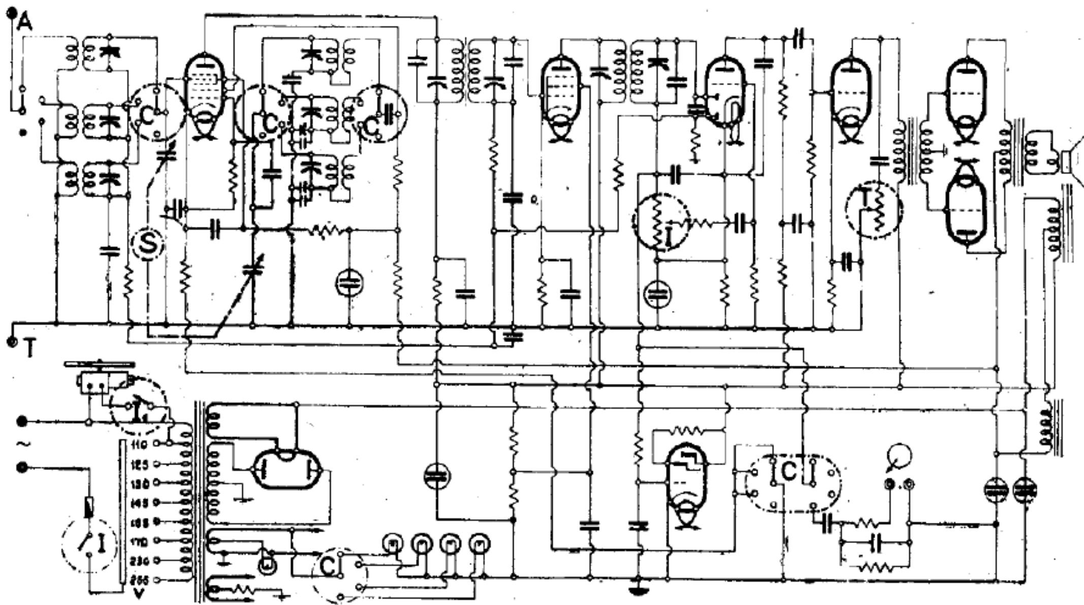
COMPAGNIA GENERALE DI ELETTRICITA' - MODD. « 252 » « 253 » « 263 »
